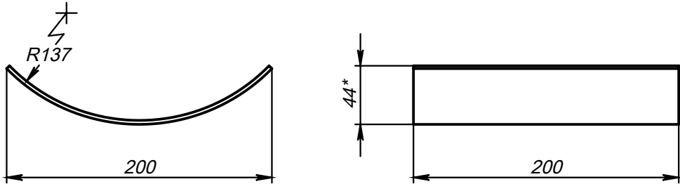
Поз.1 (Ложемент)
