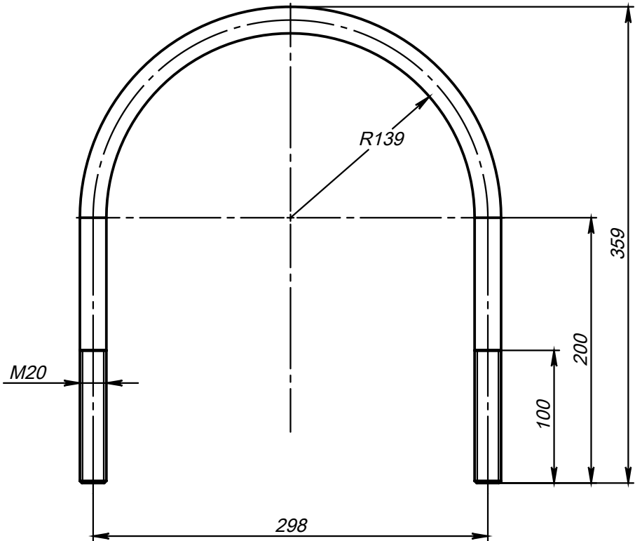
Поз.2 (Хомут)
